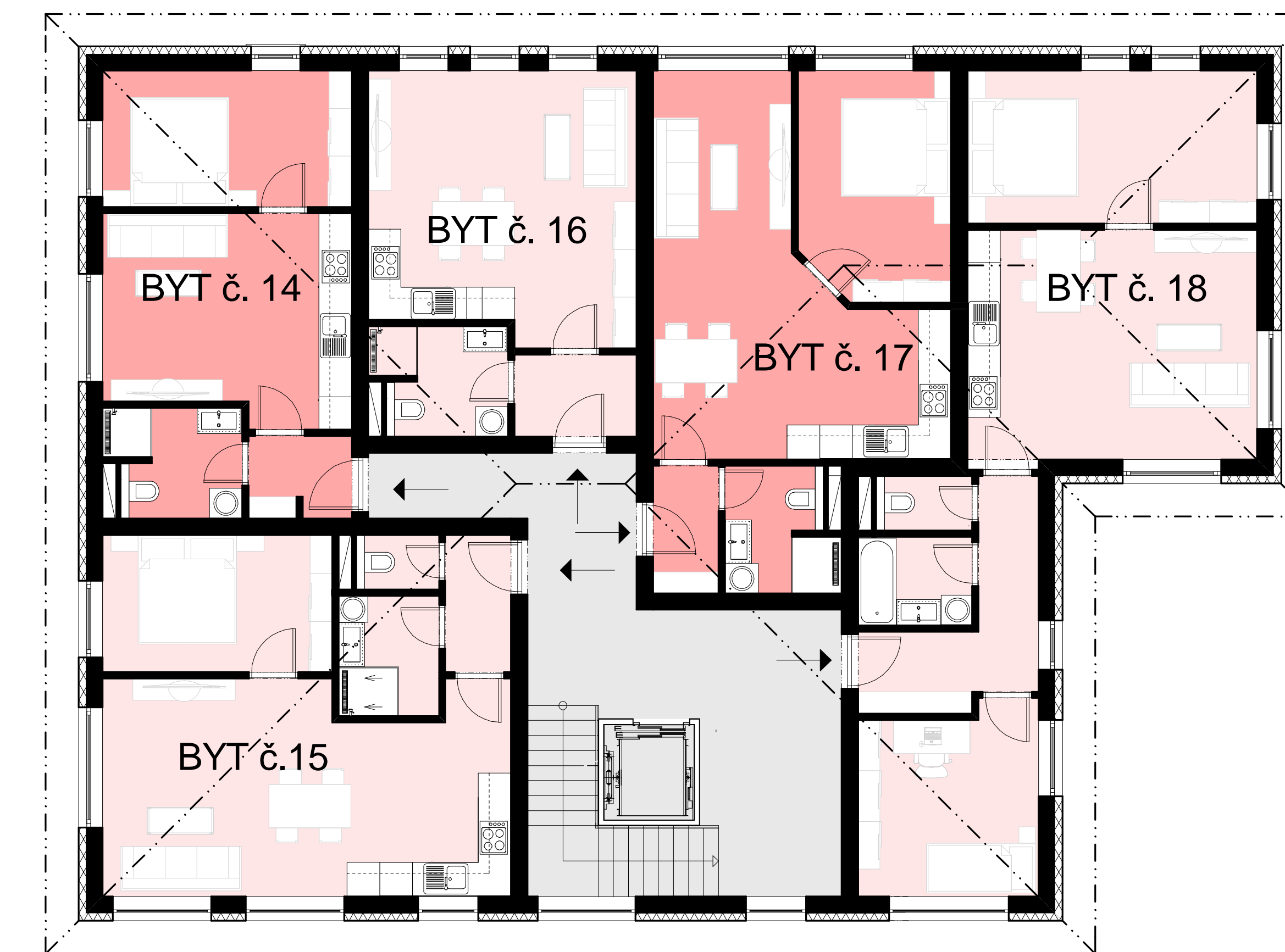
PŮDORYS 4. NP
