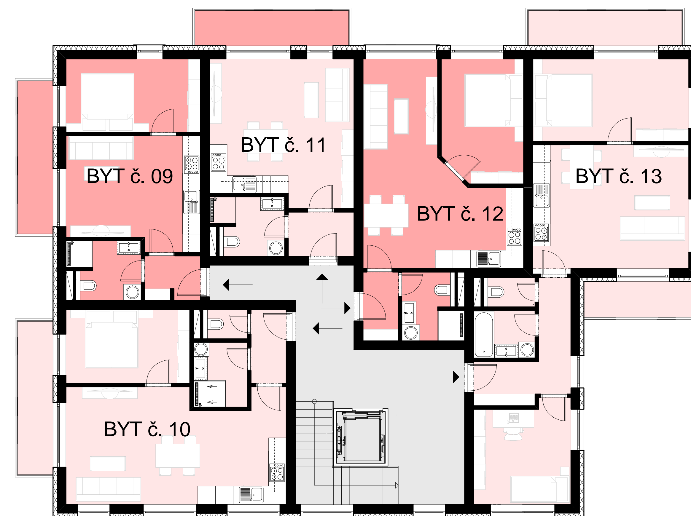
PŮDORYS 3. NP
