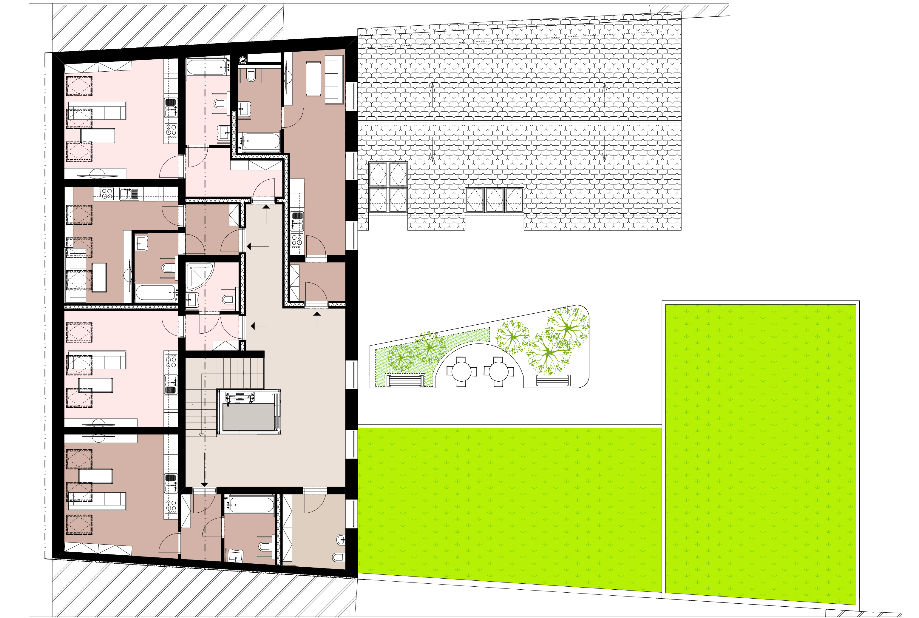
PŮDORYS 3. NP
